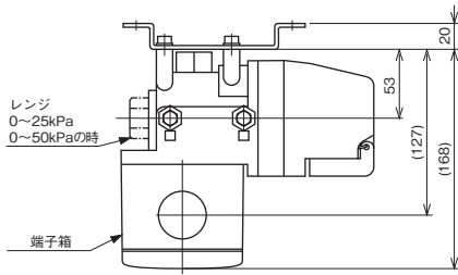
パネル取付
