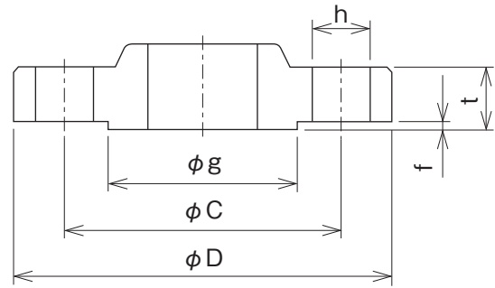
RF (平面座)
