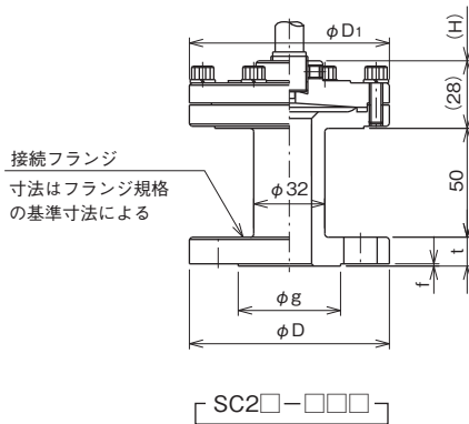
〔フランジ式〕 200形・フランジ
