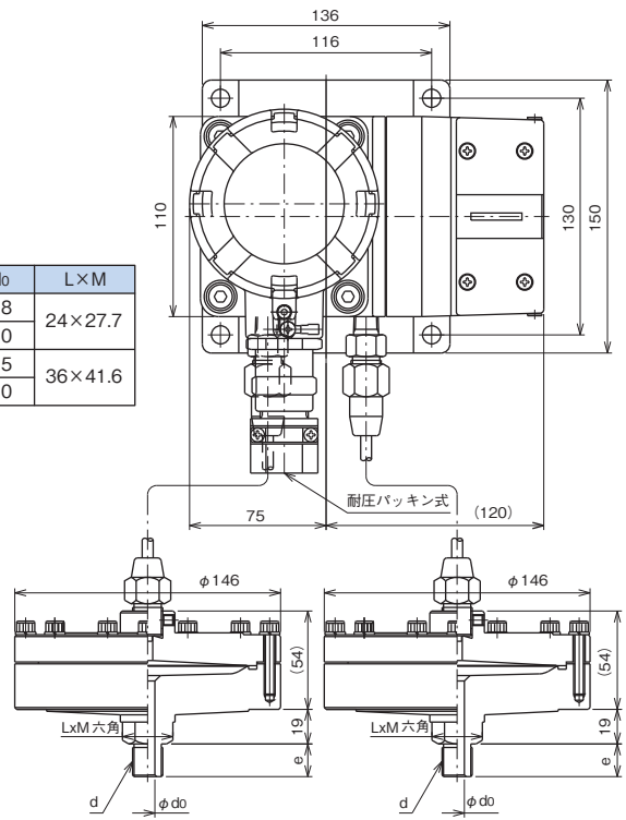
CD71 耐圧防爆形差圧カススイッチ
