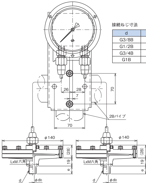
DG95・96 一般指示差圧計
