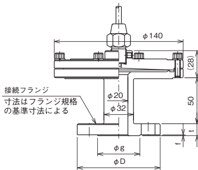
200形・フランジ
