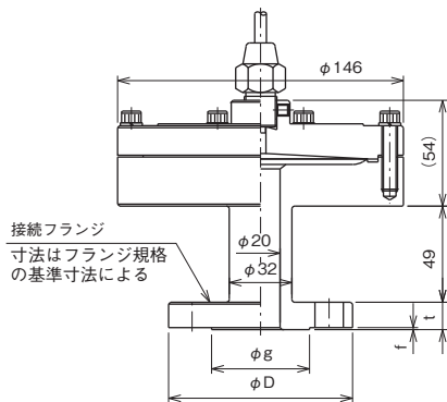
200形・フランジ
