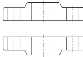
FF（全面座）
